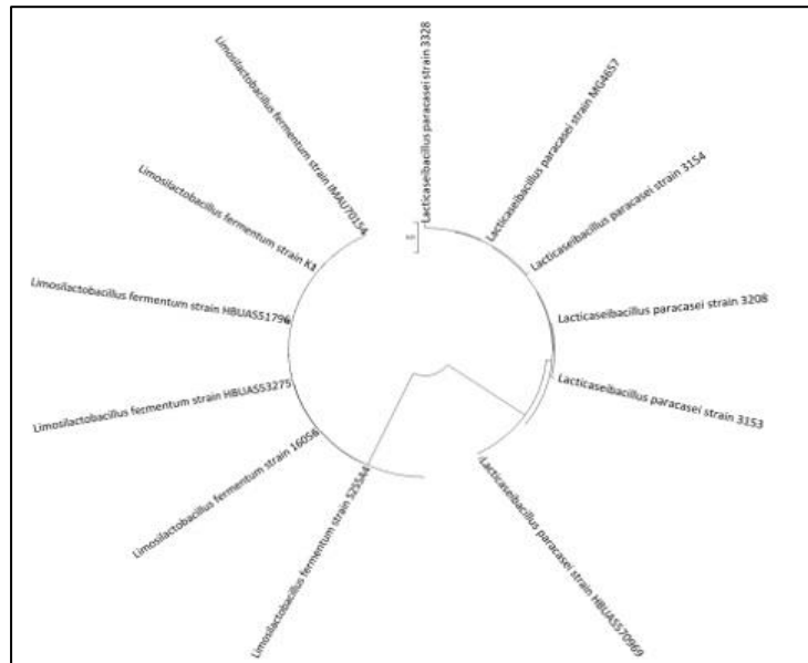
Gambar 1. Pohon filogenetik dari isolat B4, isolat B6 serta berbagai isolat Lactocaseibacillus paracasei dan Limosilactobacillus fermentum berdasarkan hasil sekuens parsial 16S rRNA. Pohon filogenetik disusun menggunakan metode Neighbor Joining dan MEGA X. Scale bar menunjukkan substitusi 0,01 per lokasi.
