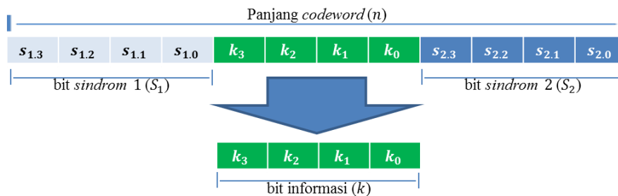
Gambar 4. Desain Decoder
