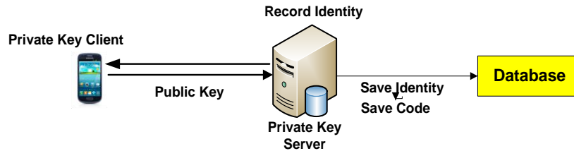
Gambar 5. Skema Pertukaran Kunci pada m-banking
