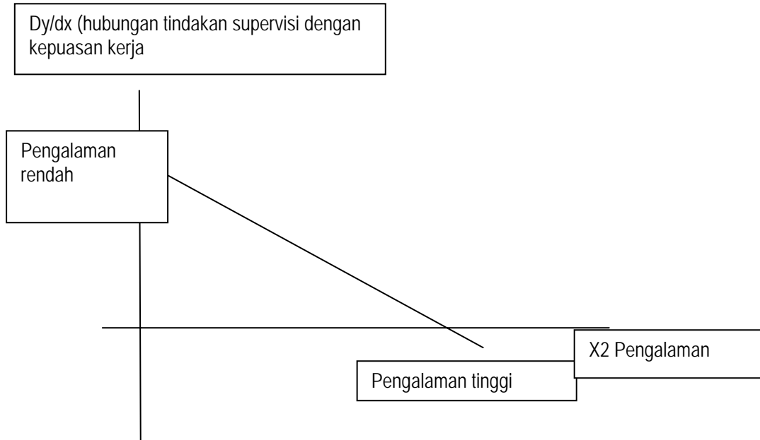
Gambar 2 Grafik Persamaan Derivatif
